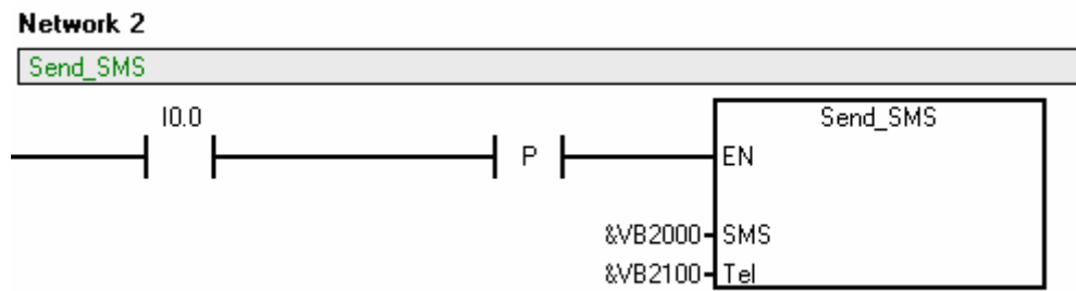
Imagen 6.2: Llamada a la función Send_SMS
