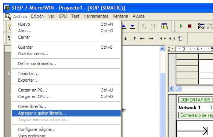
Imagen 4.1: Agregar librería
